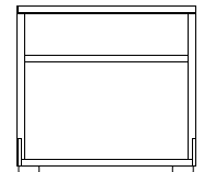
Edison Night Stand EDI-O32 18W x 16D x 24H EDI-O43 18W x 16D x 28H EDI-O49 24W x 16D x 24H EDI-O45 24W x 16D x 28H
